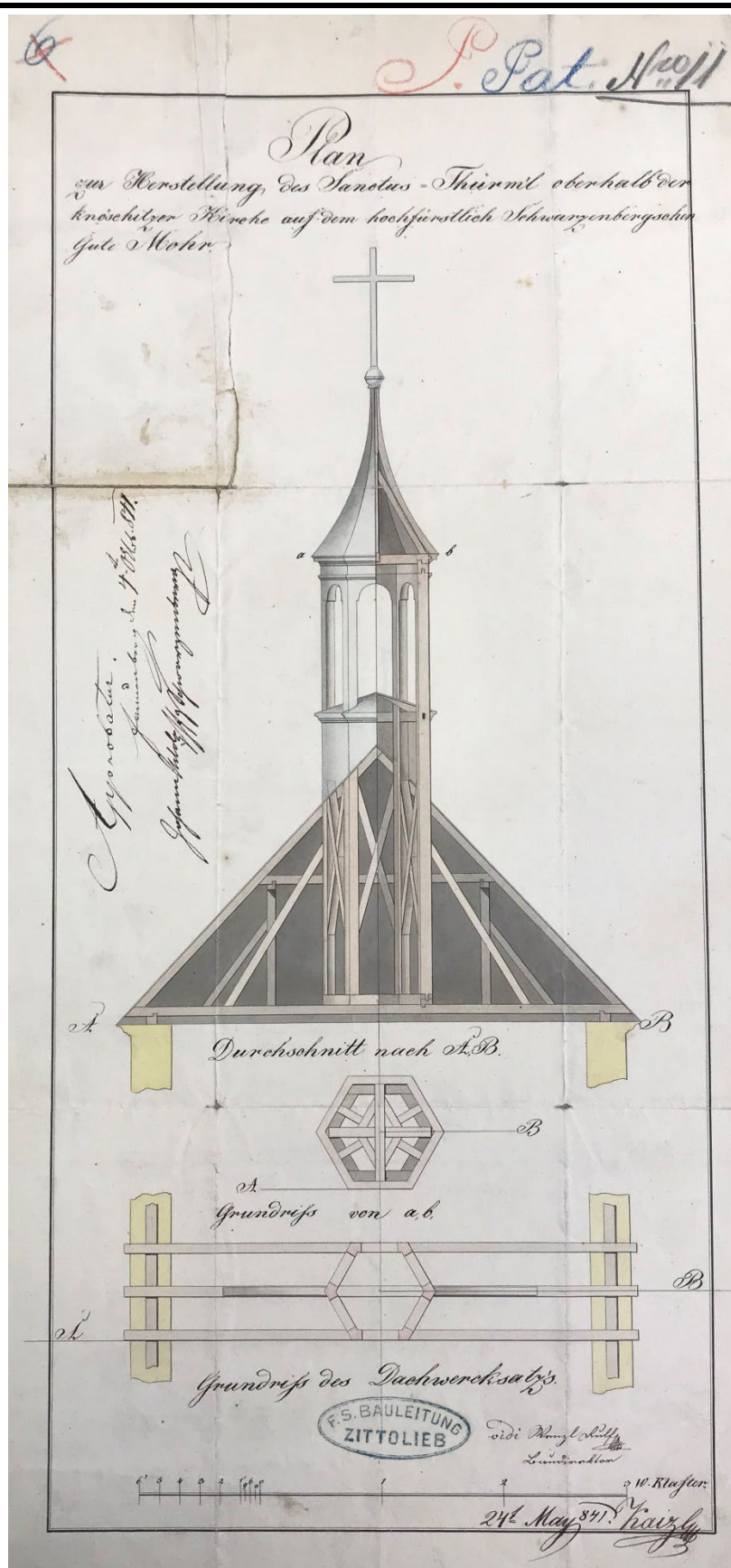
Stavební plán na stavbu sanktusníkové věže od schwarzenberského stavitele Kaizla z roku 1841. (SOA Třeboň, Velkostatek Postoloprty, plány – nezpracováno)
